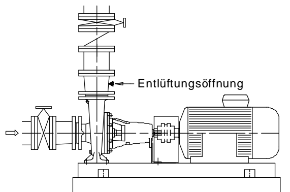
Auffüllung einer Pumpe unter Druck
