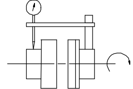
Mit einer Meßuhr
