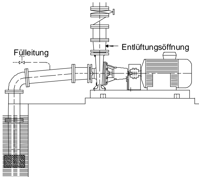
Auffüllen einer Pumpe in Saugbetrieb mit Fußventil
