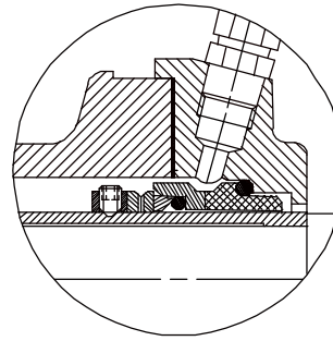
Einfache Gleitringdichtung Andere Pumpen ME
