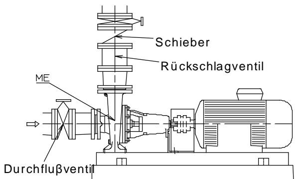
Pumpe mit Zulauf
