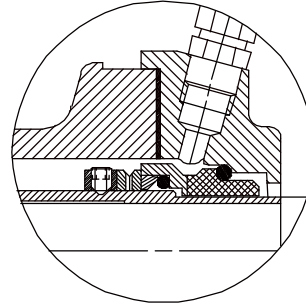
Entlastete Gleitringdichtung Andere Pumpen ME
