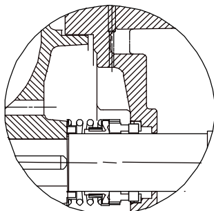
Gleitringdichtung Für ME 150-200, 200-250, 200-315 200-355, 250-250 250-315, 300-300
